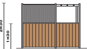
PORTE COULISSANTE SANS BARREAUDAGE SUPÉRIEUR, À L'EXCEPTION DU BARREAU RÉTRACTILE D'OUVERTURE ET D'UN BARREAU DE PROTECTION
