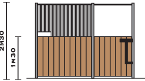
PORTE À 1 VANTAIL SANS BARREAUDAGE PARTIE FIXE AVEC BARREAUDAGE SUPÉRIEUR VERTICAL ET LUCARNE D'AFFOURAGEMENT
