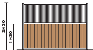
PARTIE BASSE PLEINE ET PARTIE SUPÉRIEURE AVEC BARREAUDAGE VERTICAL
