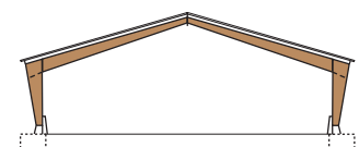
Fermes portiques, 3 articulations Poteaux renversés
