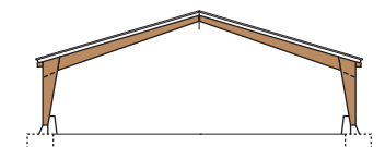
Fermes portiques, 3 articulations
